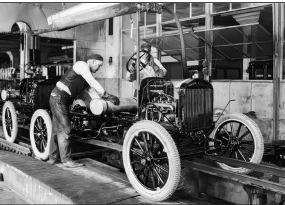
Конвеєр на заводі Г. Форда. Початок XX ст.
