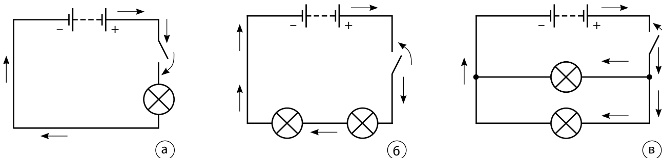
Мал. 4.3. Приклади електричних схем: схема ліхтарика (а); послідовне з'єднання споживачів (б); паралельне з'єднання споживачів (в)
