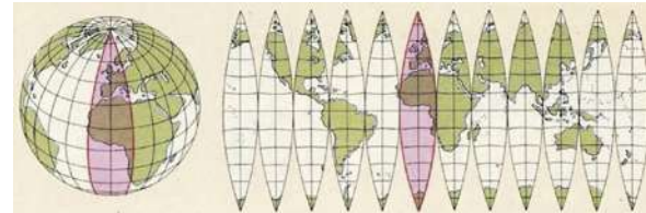
Мал. 3.15. Проекція глобуса на площині — це приклад розгортки сфери
