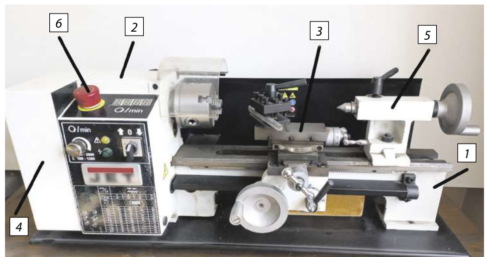
Мал. 14.3. Основні вузли токарно-гвинторізного верстата
