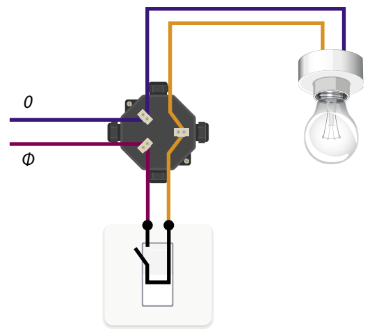
Мал. 4.5. Електрична схема підключення світильника
