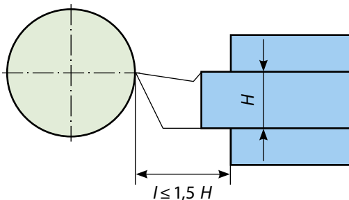
Мал. 14.7. Установлення різця
