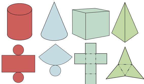
Мал. 3.1. Розгортки деяких геометричних фігур
