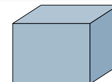
Прямокутний паралелепіпед
