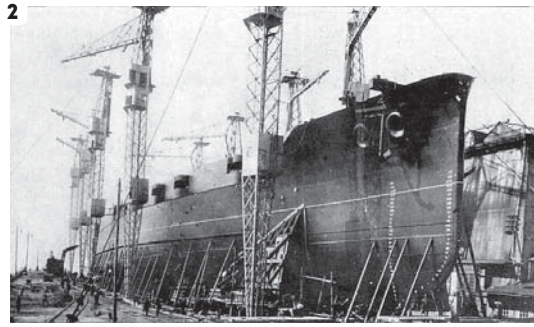
2 — Будівництво пароплава на Миколаївському заводі. 1914 р.
