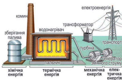
Мал. 96. Теплова генерація електроенергії https://cutt.ly/8tRomWS0
