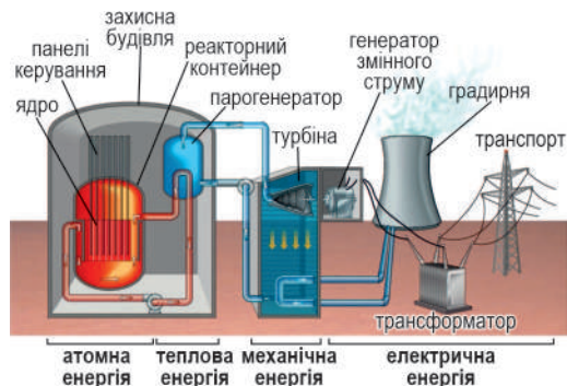
Мал. 97. Атомна генерація електроенергії https://cutt.ly/8tRomWS0
