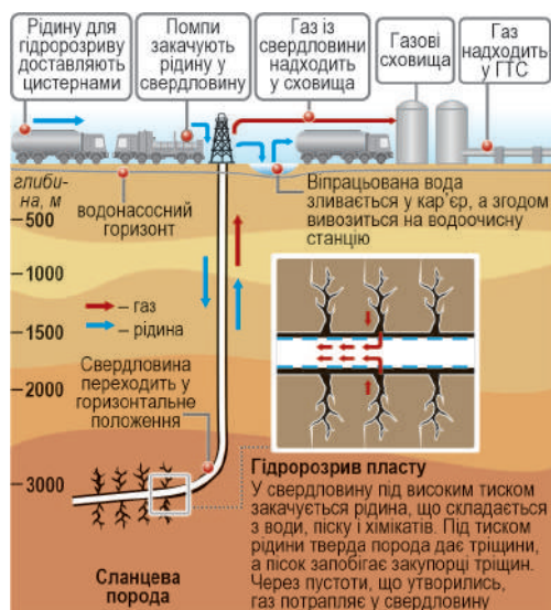
Мал. 81. Схема видобутку сланцевого газу
