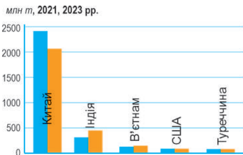
Мал. 115. Найбільші виробники цементу
