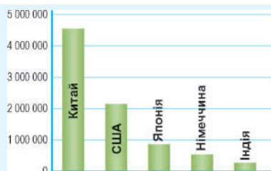
Мал. 121. Загальна продукція машинобудування, млн дол., 2024 р.
