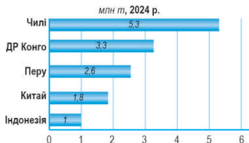
Мал. 91. Країни з найбільшим видобутком міді
