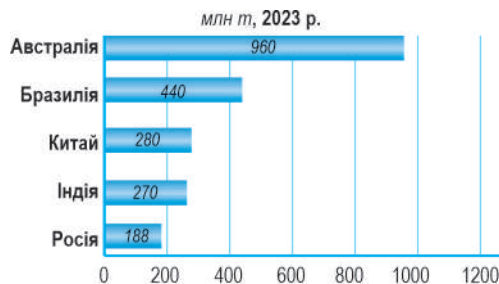
Мал. 86. Країни з найбільшим видобутком залізних руд
