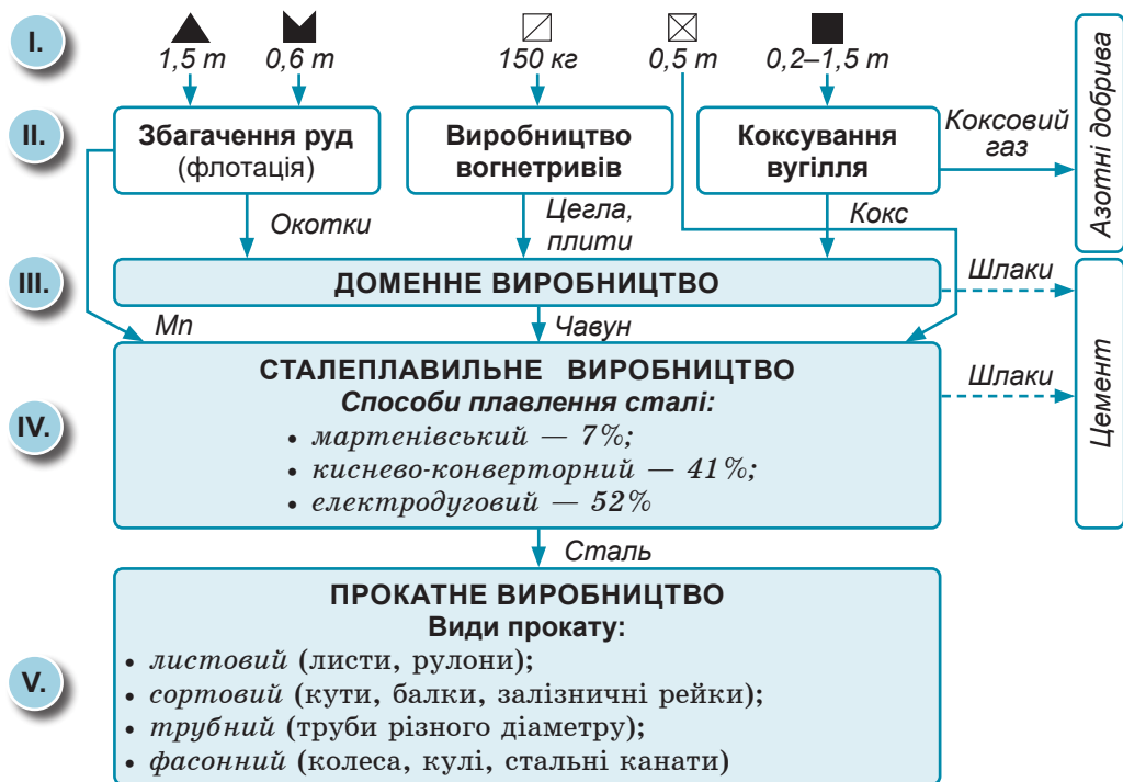
Мал. 114. Комбінат із повним металургійним циклом
