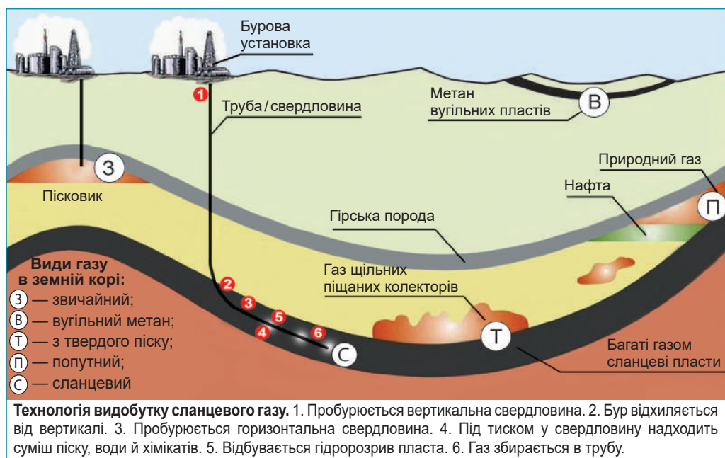
Мал. 83. Схема залягання та видобутку сланцевого газу
