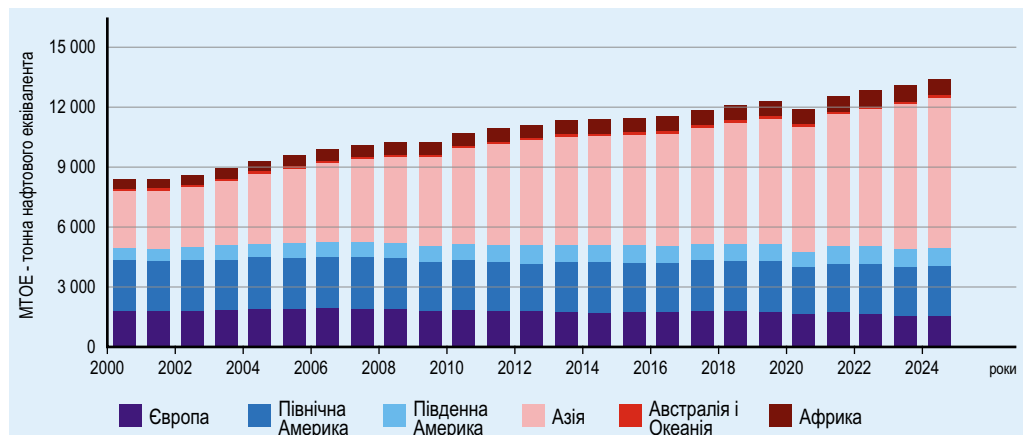
Мал. 18.2. Динаміка енергоспоживання у світі, 2000–2024 рр.
