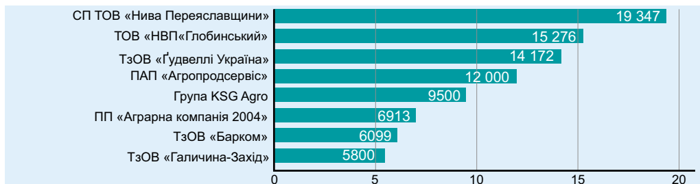
Мал. 15.5. Найбільші (за поголів'ям) свиногосподарства України, тис. голів, 2024 р.
