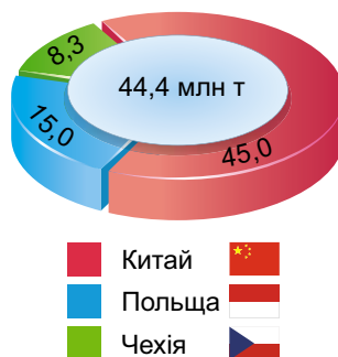
Мал. 16.12. Експорт залізорудної сировини України, % від ваги, 2024 р.
