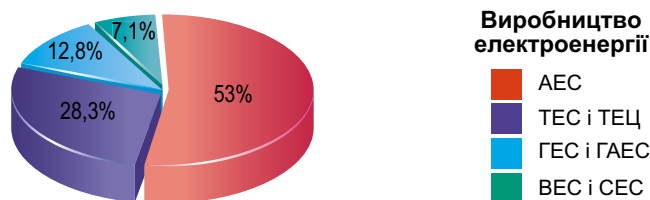
Мал. 18.5. Обсяг виробництва електроенергії в Україні, млн кВт · год, 2024 р.
