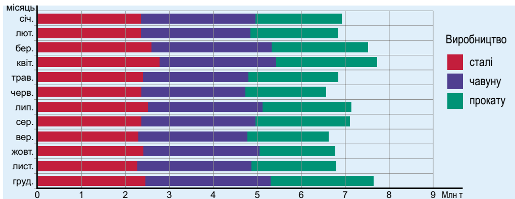
Мал. 20.3. Обсяг виробництва основної продукції ПАТ «Запоріжсталь», млн т, 2024 р.
