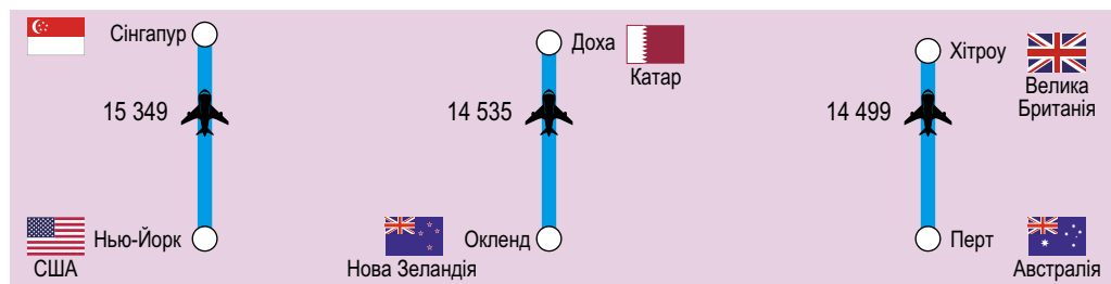
Мал. 39.10. Найдовші регулярні безпересадкові пасажирські комерційні авіарейси, км
