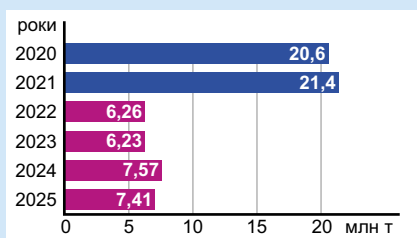
Виробництво сталі 2020–2025 рр.
