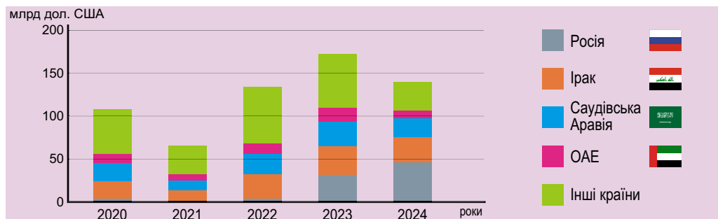
Мал. 39.6. Країни-лідери з імпорту сирової нафти до Індії, млрд дол. США, 2020–2024 рр.
