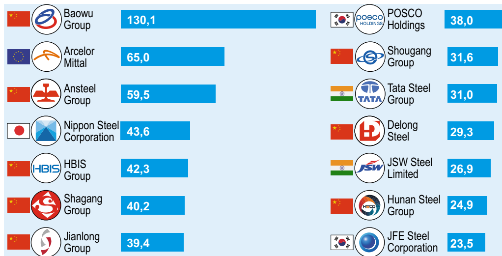
Мал. 19.6. Провідні компанії з виробництва сталі у світі, млн т, 2024 р.
