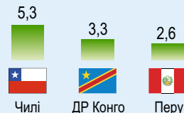
Мал. 16.8. Країни-лідери з видобування руд металів у світі, млн т, 2023 р.
