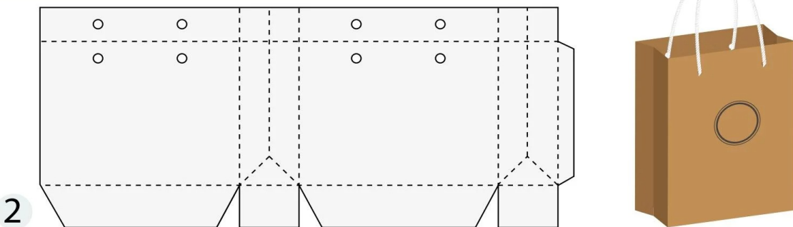
Розгортка пакування для тістечок
