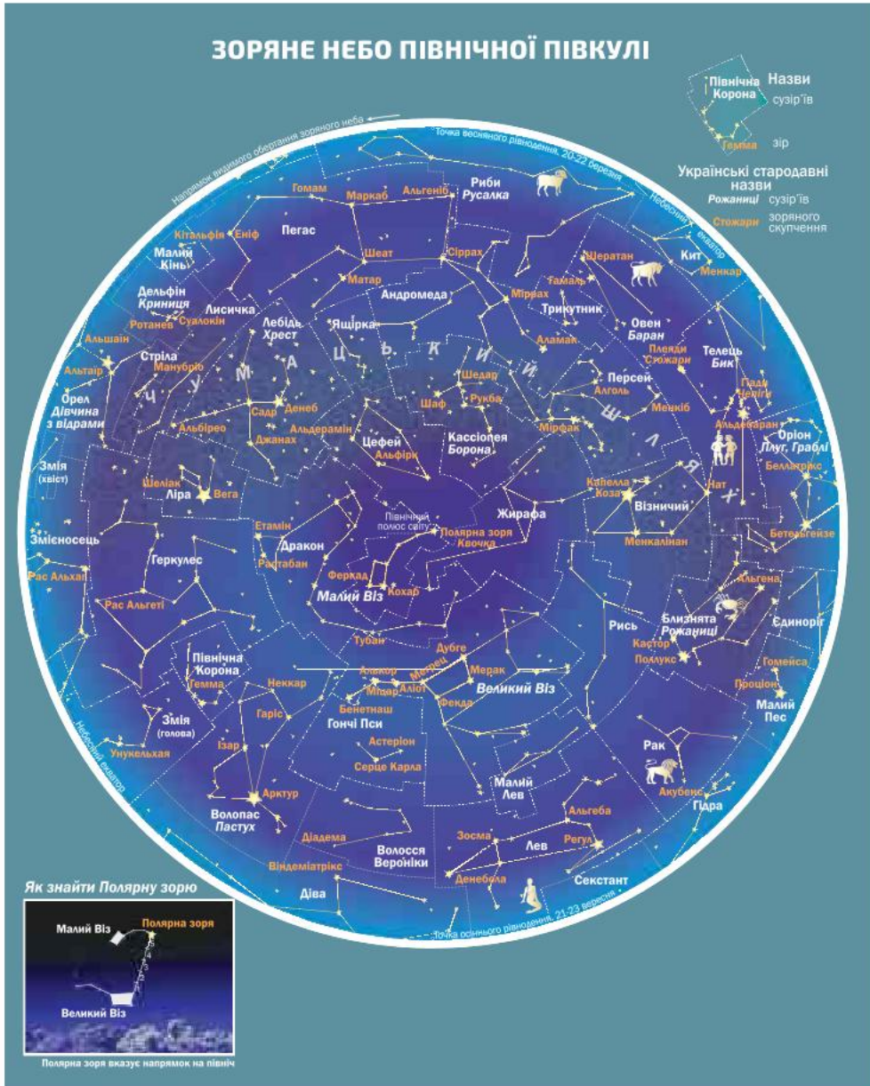
Карта зоряного неба Північної півкулі Землі
