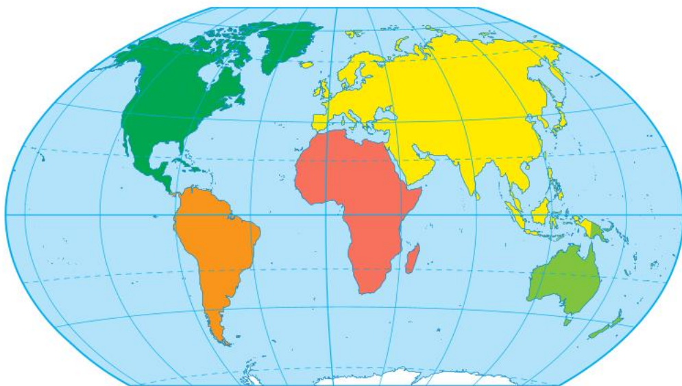
Карта материків та океанів
