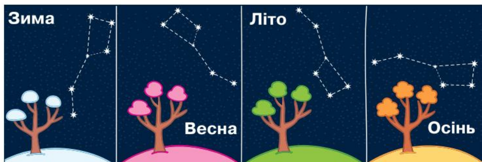
Сузір'я Великий Віз у різні пори року
