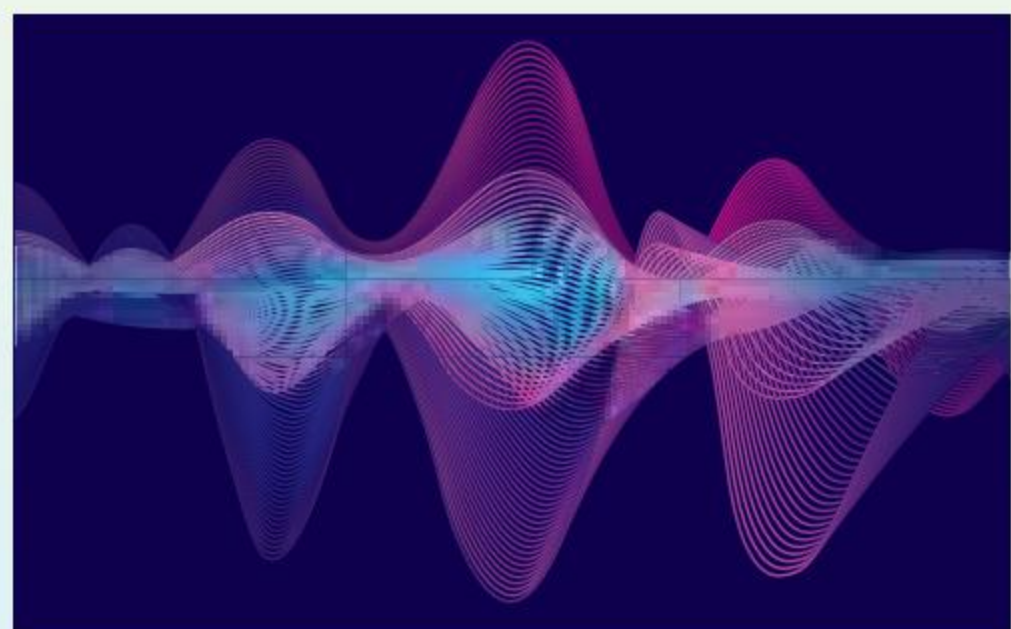
Зображення звукової хвилі
