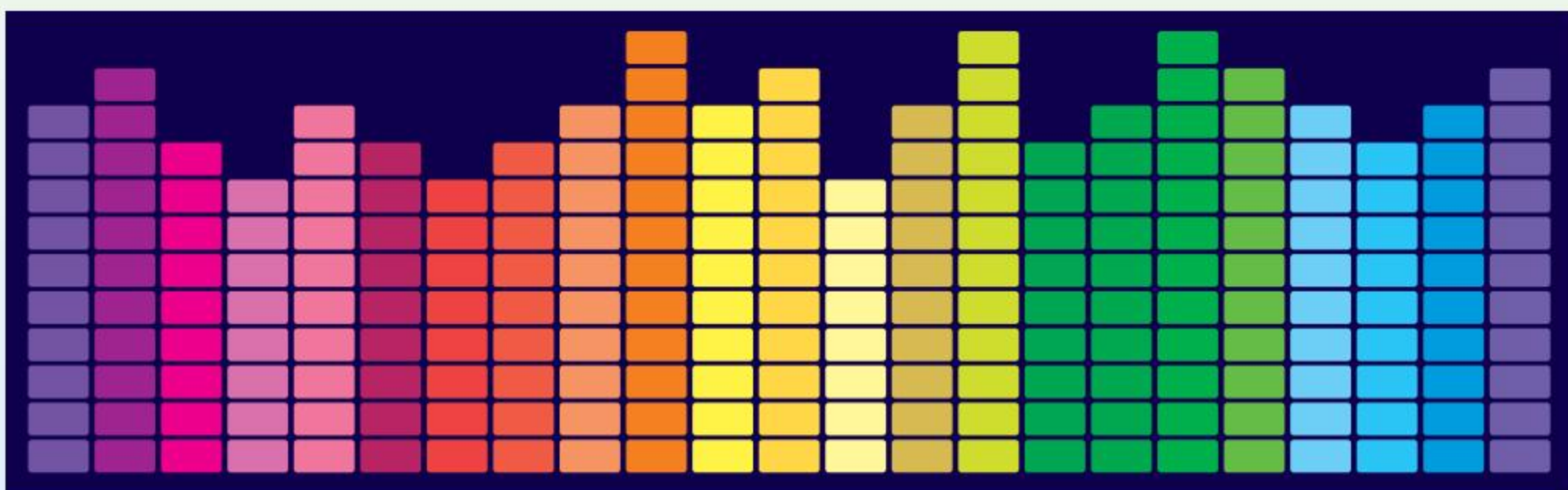
Зображення звука в музичному еквайзері
