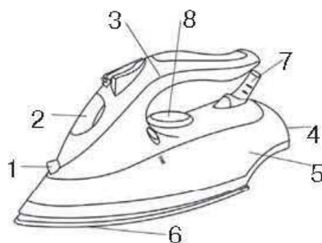
Мал. 36. Загальна будова праски: 1 — розбризкувач; 2 — отвір для наповнення водою; 3 — ручка праски; 4 — п’ятка праски; 5 — резервуар для води; 6 — підшва праски; 7 — шарнір для захисту шнура від перекручування; 8 — терморегулятор
