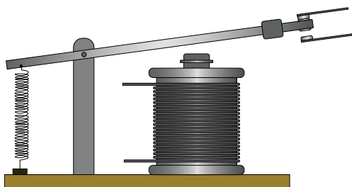
Рис. 10.20. Електромагнітне реле
