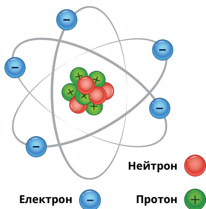
Рис. 4.10. Модель атома Бора
