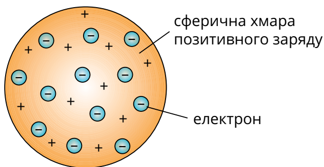
Рис. 4.6. Модель Томсона, відома як «сливовий пудинг», названа за аналогією зі старовинним англійським пудингом зі сливами
