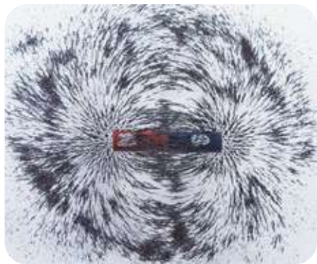
Рис. 10.5. Лінії магнітного поля
