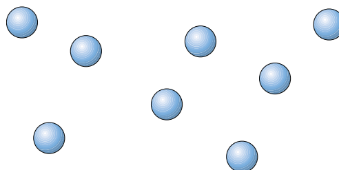
Рис. 4.3. Модель атома Дальтона
