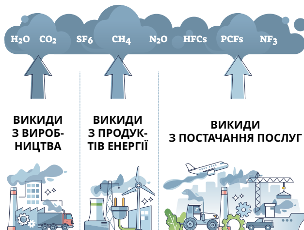
Рис. 11.17. Основні парникові газу
