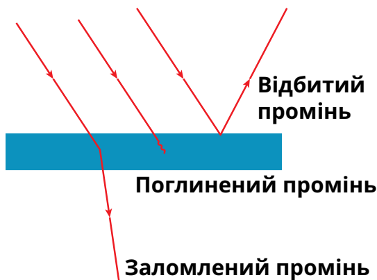
Рис. 9.12. Заломлення, поглинання та відбивання світлового променя
