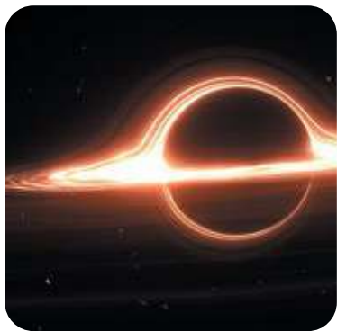
Рис. 13.12. Чорна діра
