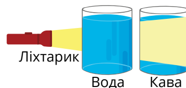
Рис. 9.31. Дослідження прямолінійного поширення світла
