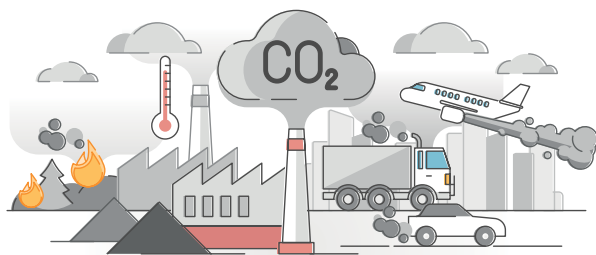
Рис. 11.18. Викиди вуглекислого газу \text{CO}_2
