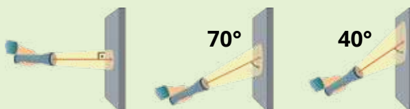
Рис. 9.10. Промінь світла, що падає на поверхню під різними кутами
