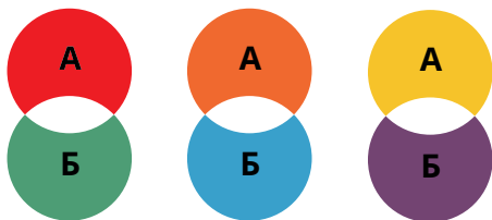
Рис. 9.25. Доповняльні кольори
