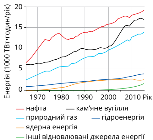
Рис. 12.22. Світове енергоспоживання з 1965 року
