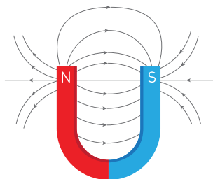
Рис. 10.7. Силові лінії магнітного поля підковоподібного магніту
