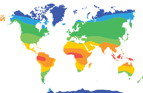
Рис. 11.8. Карта кліматичних поясів
