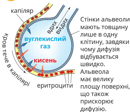
Рис. 1.14. Газообмін в альвеолі
