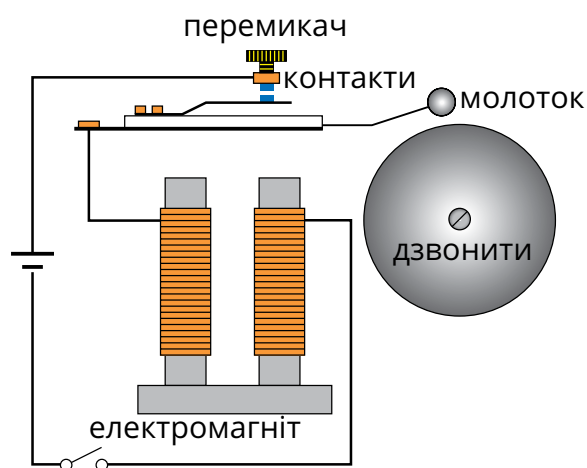
Рис. 10.23. Схема електричного дзвоника
