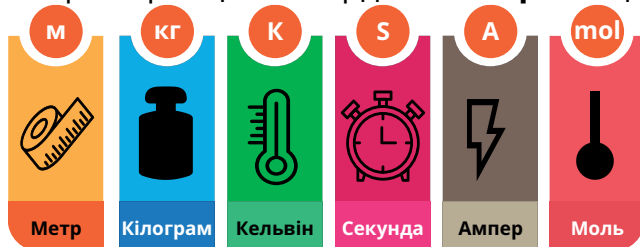
Рис. 7.4. Основні одиниці системи СІ
