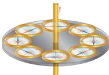
Рис. 10.15. Стрілки компаса орієнтуються вздовж ліній магнітного поля
