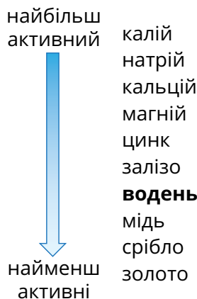
Рис. 6.27. Ряд активності деяких металів
