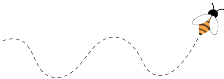
Рис. 7.1. Траєкторія руху бджоли
