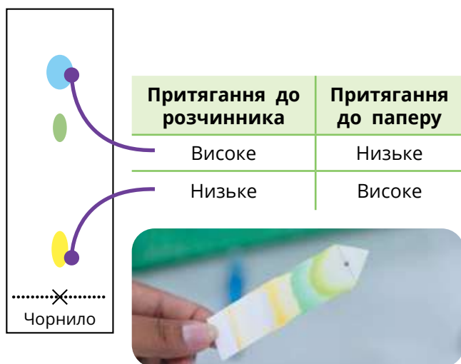
Рис. 4.16. Положення барвника залежить від його притягання до розчинника та паперу
