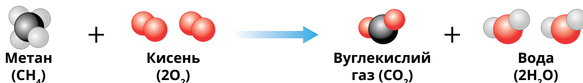
Рис. 6.6. Графічна та текстова схеми горіння метану
