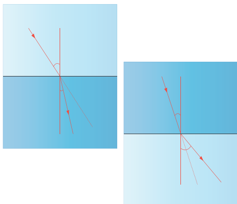
Рис. 9.14. Текстова формула другого закону заломлення світла
