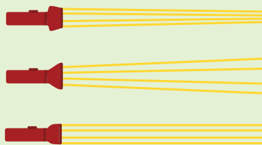
Рис. 9.5. Світлові пучки
