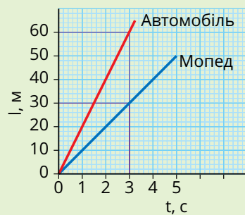
Рис. 7.13. Графіки руху автомобіля та мопеда
