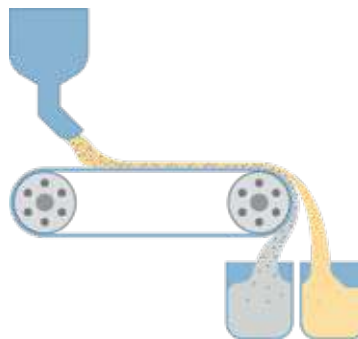
Рис. 10.22. Схема магнітного сепаратора
