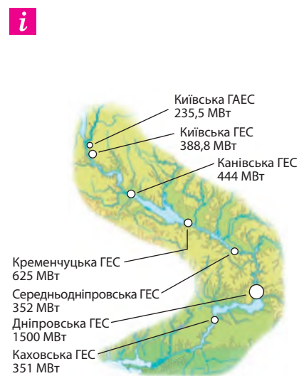
Мал. 2. Каскад ГЕС на Дніпрі.
