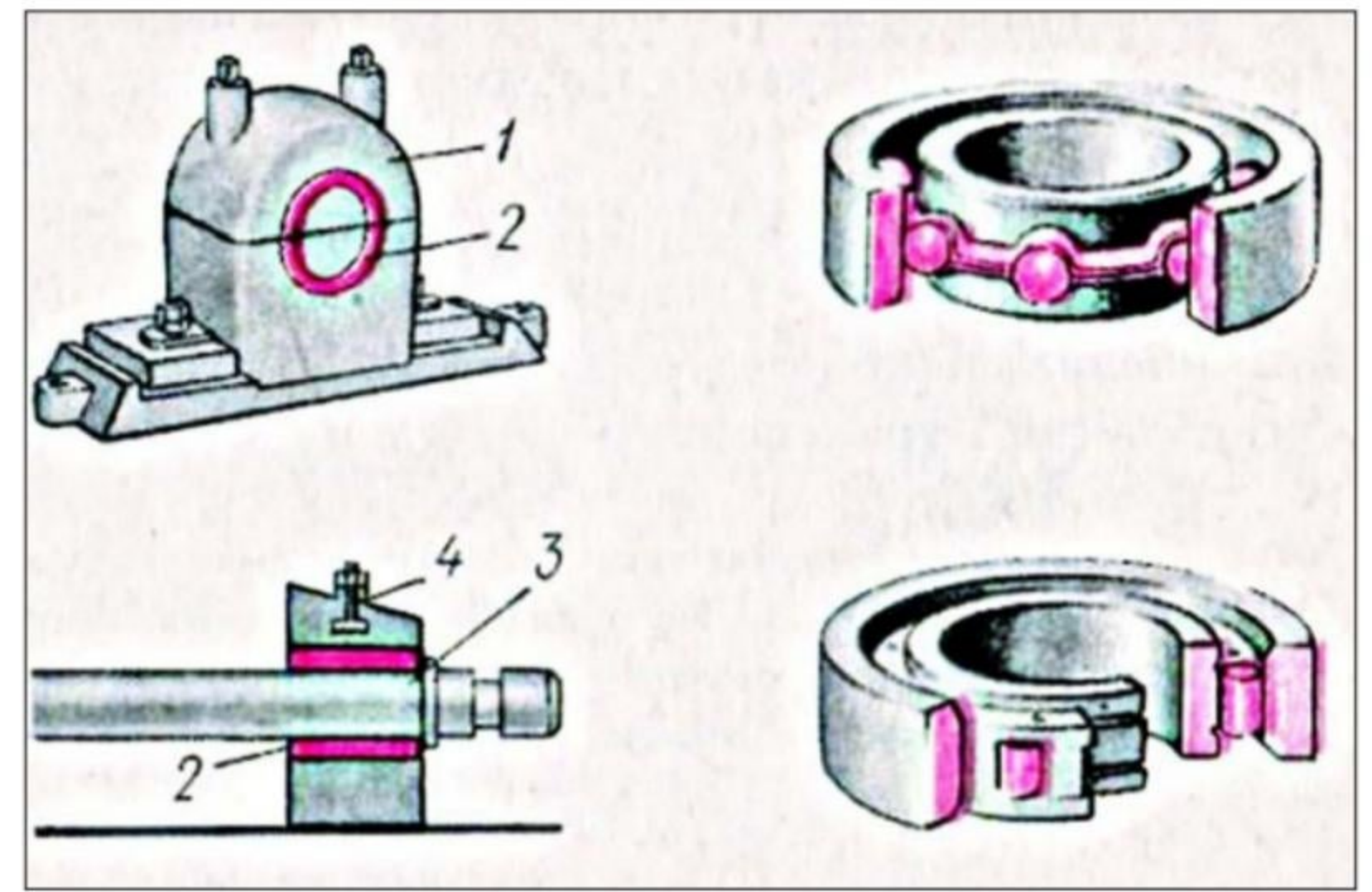
Мал. 91. Підшипники ковзання: 1 — корпус підшипника; 2 — вкладиш; 3 — вал; 4 — отвір для змащування
