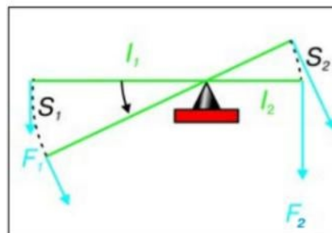
Мал. 130. Важіль не дає виграшу в роботі
