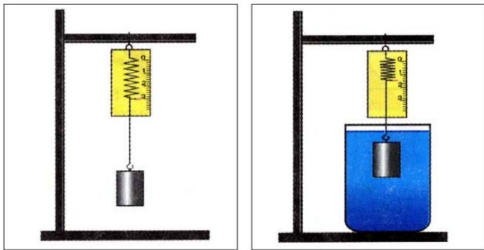
Мал. 104. Прилади для визначення густини твердого тіла.
