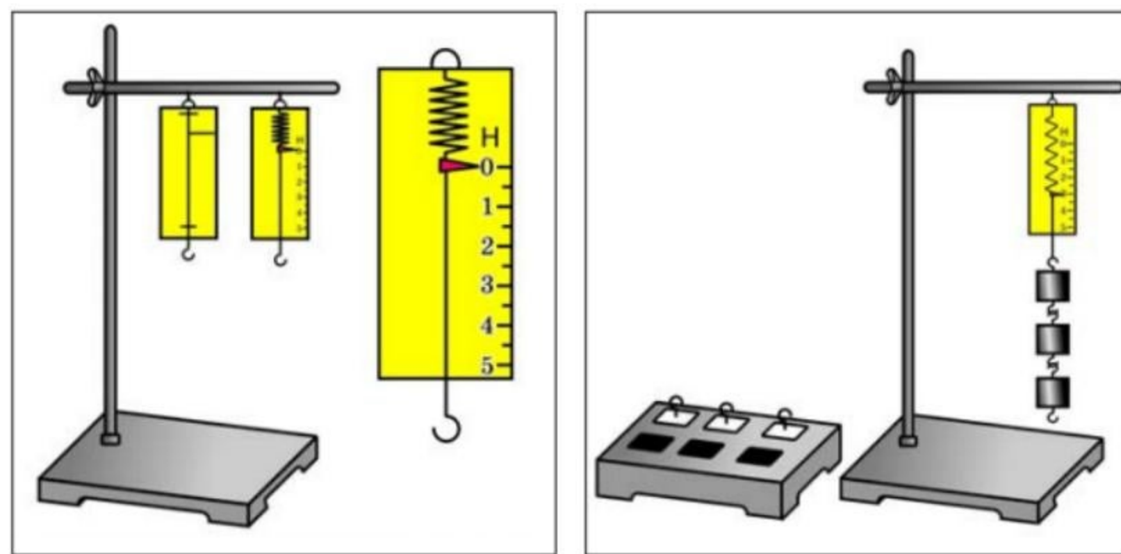
Мал. 73. Прилади до лабораторної роботи №8
