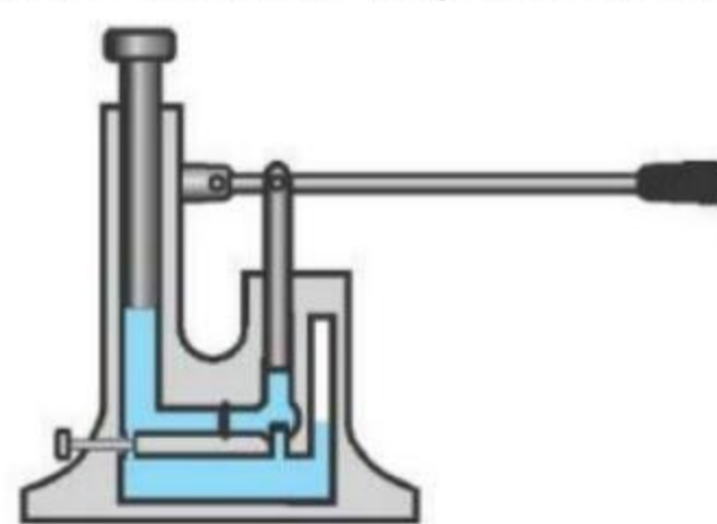
Мал. 122. До задачі 3
