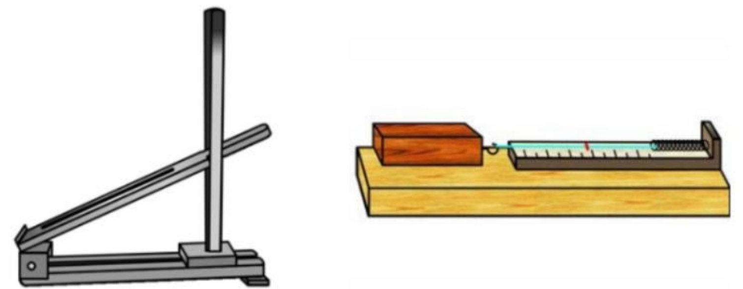
Мал. 129. Прилади до лабораторної роботи
