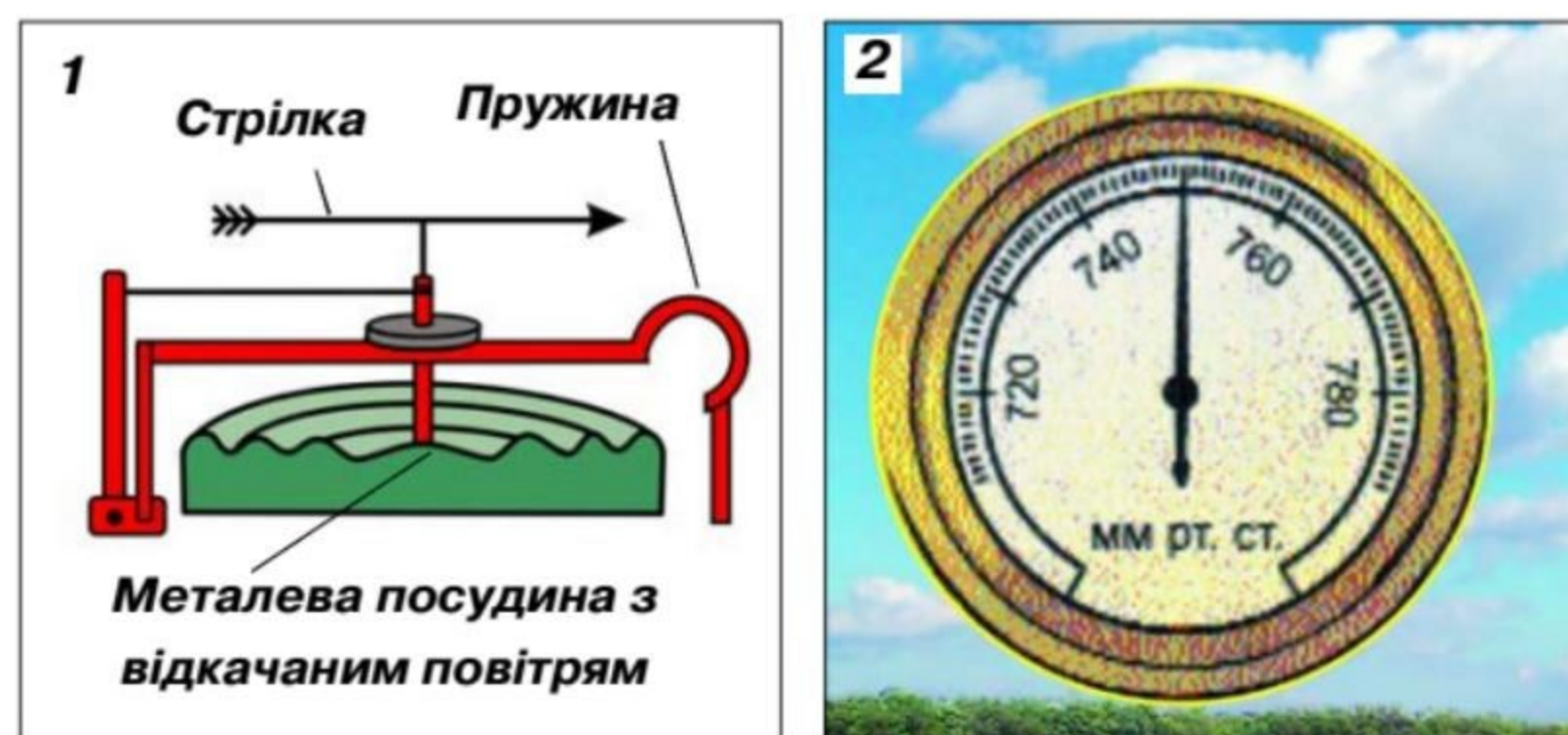
Мал. 102. Будова (1) та зовнішній вигляд (2) барометра-анероїда
