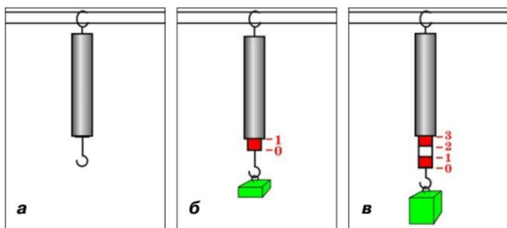
Мал. 74. Градування динамометра
