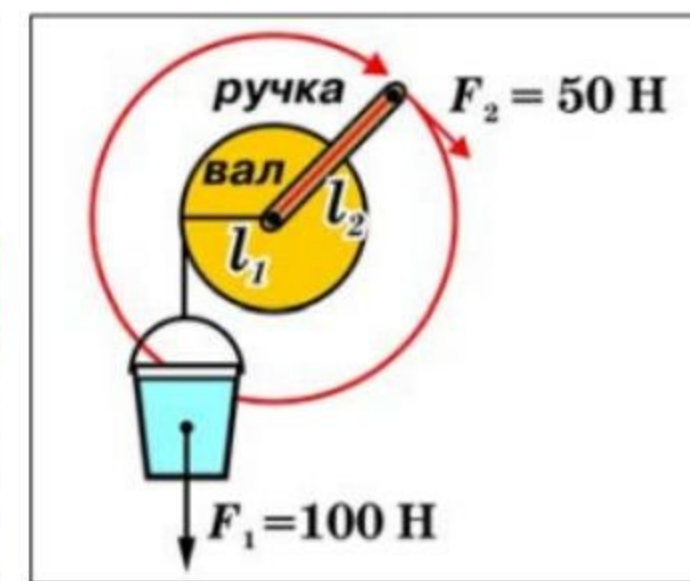
Мал. 116. Коловорот
