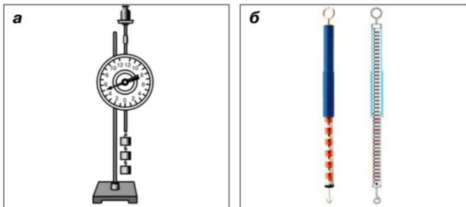
Мал. 72. Динамометри: а — демонстраційний; б — трубчастий (будова)
