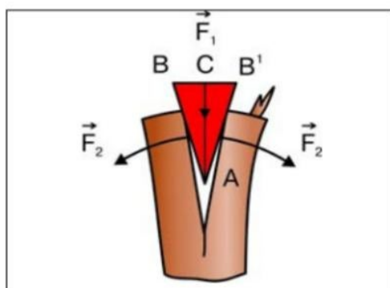
Мал. 120. Клин дає виграш у силі
