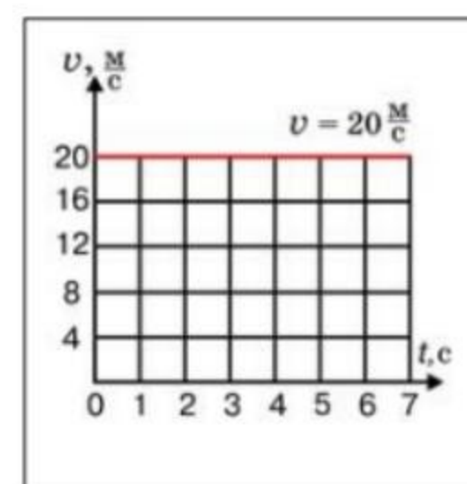
Мал. 38. До задачі 4
