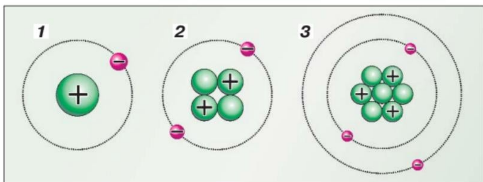
Мал. 8. Моделі атомів: 1 — Гідрогену; 2 — Гелію; 3 — Літію
