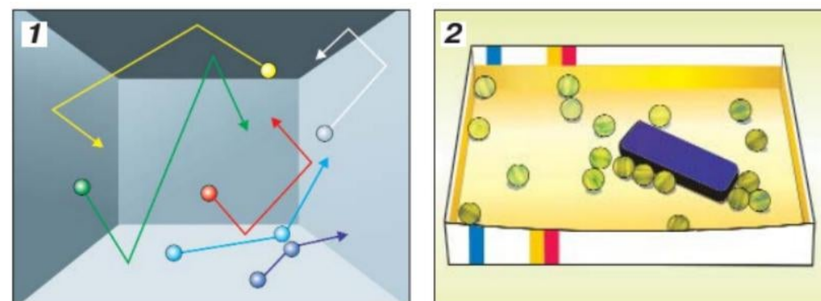
Мал. 14. Моделі броунівського руху частинок
