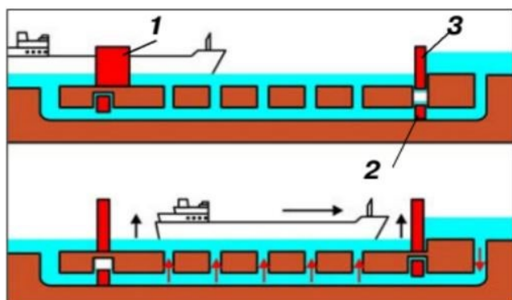
Мал. 97. Річковий шлюз в сполучених посудинах
