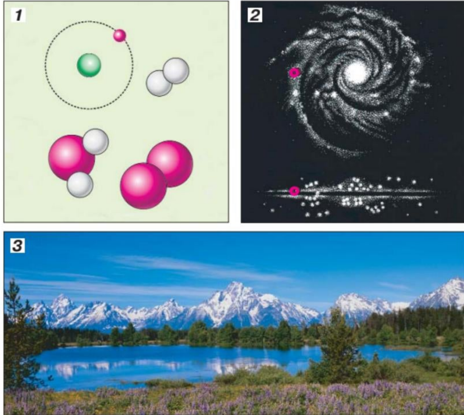
Мал. 3. 1 — атом, молекули; 2 — вигляд нашої Галактики з космічного простору (червоним обведене місцезнаходження Сонячної системи); 3 — об'єкти макросвіту
