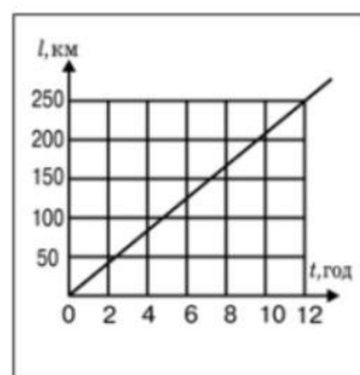
Мал. 36. До задачі 2
