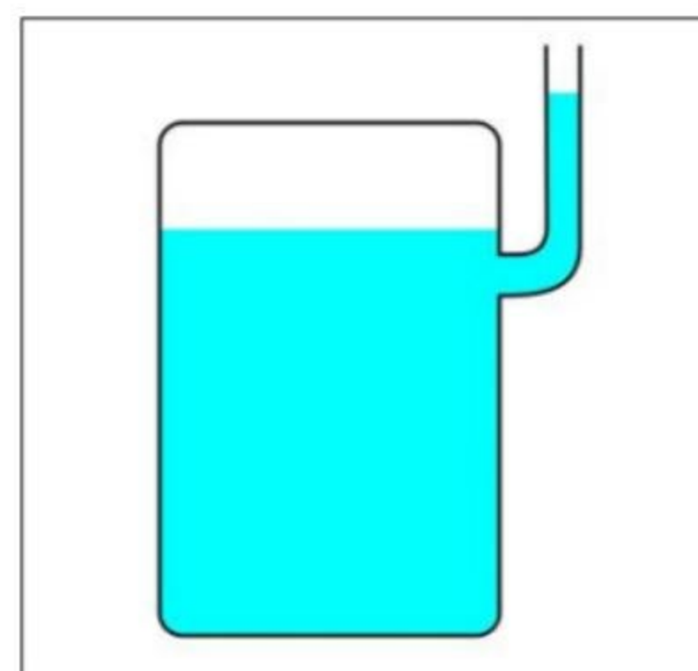
Мал. 101. До задачі 3
