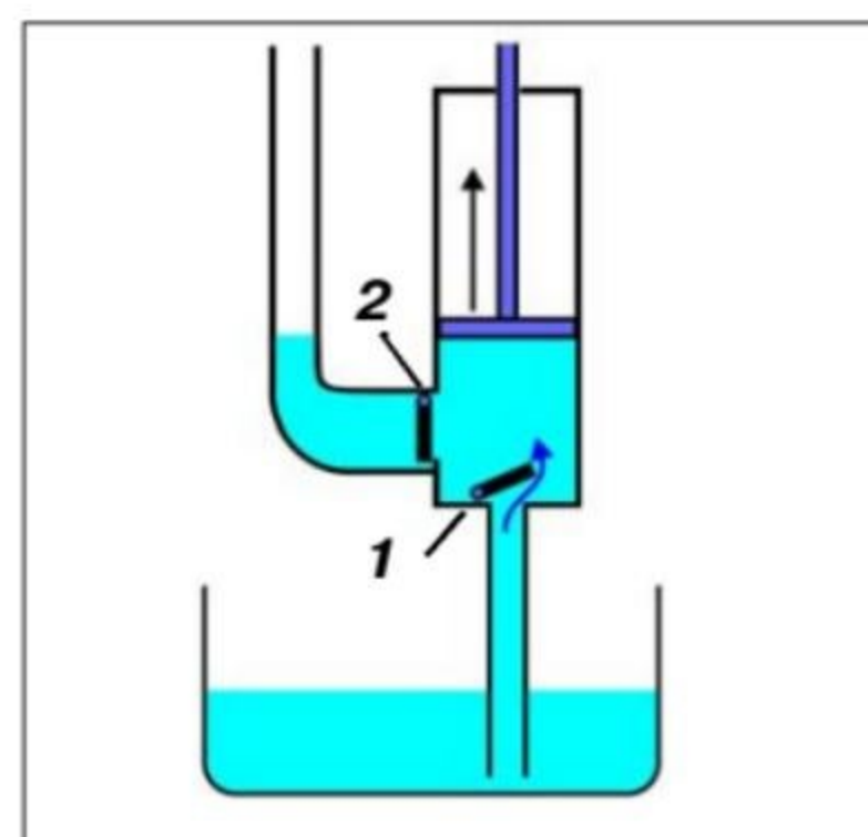
Мал. 100. Рідинний насос
