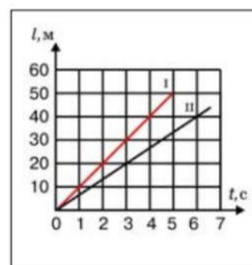
Мал. 37. До задачі 3
