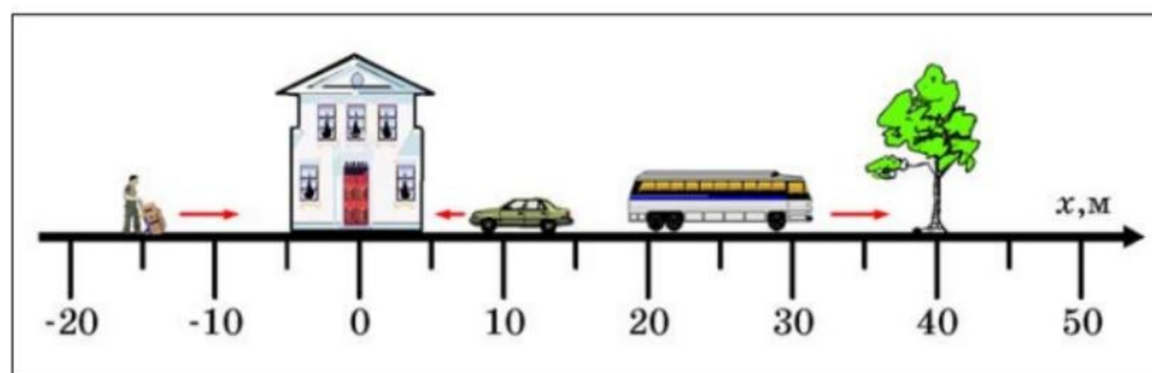
Мал. 27. Розташування об'єктів відносно тіла відліку
