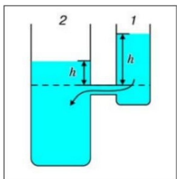
Мал. 96. Схема руху рідини
