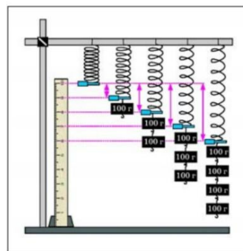
Мал. 62. Маса — міра гравітаційних властивостей тіла
