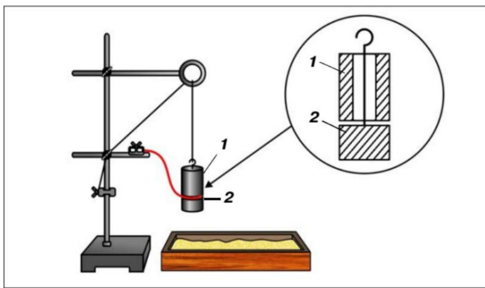
Мал. 87. Демонстрування невагомості тіла
