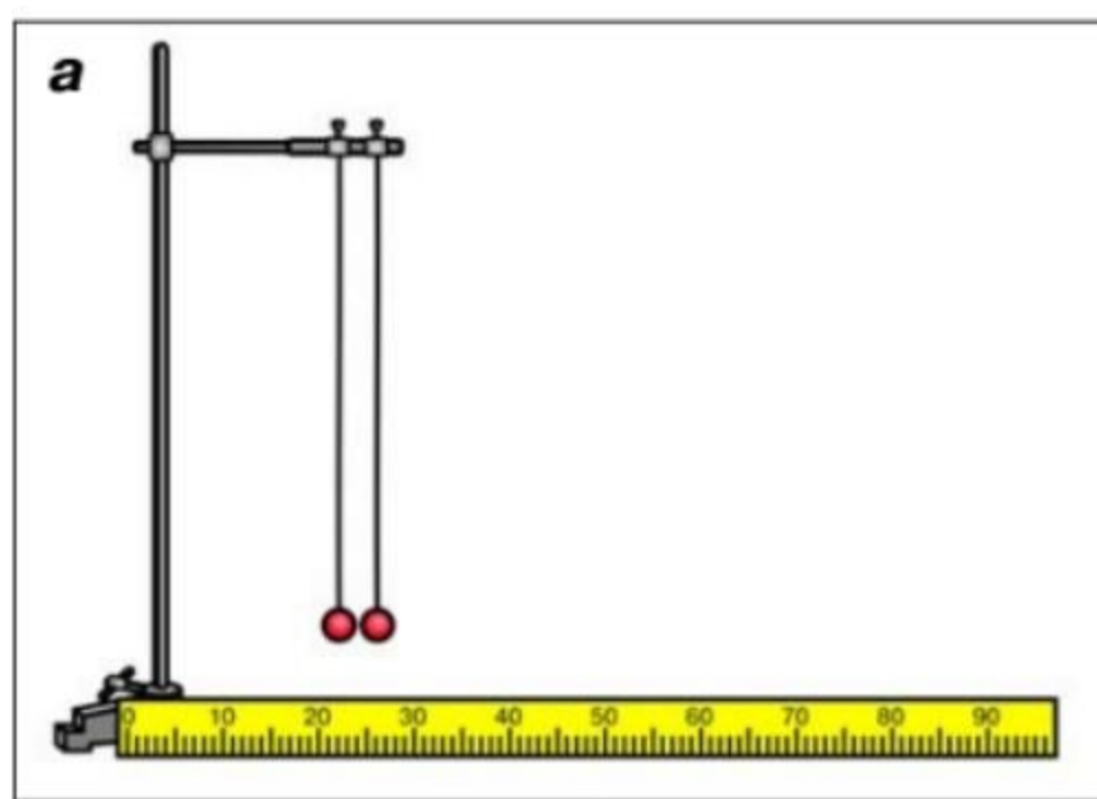
Мал. 48. Прилади до лабораторної роботи № 5
