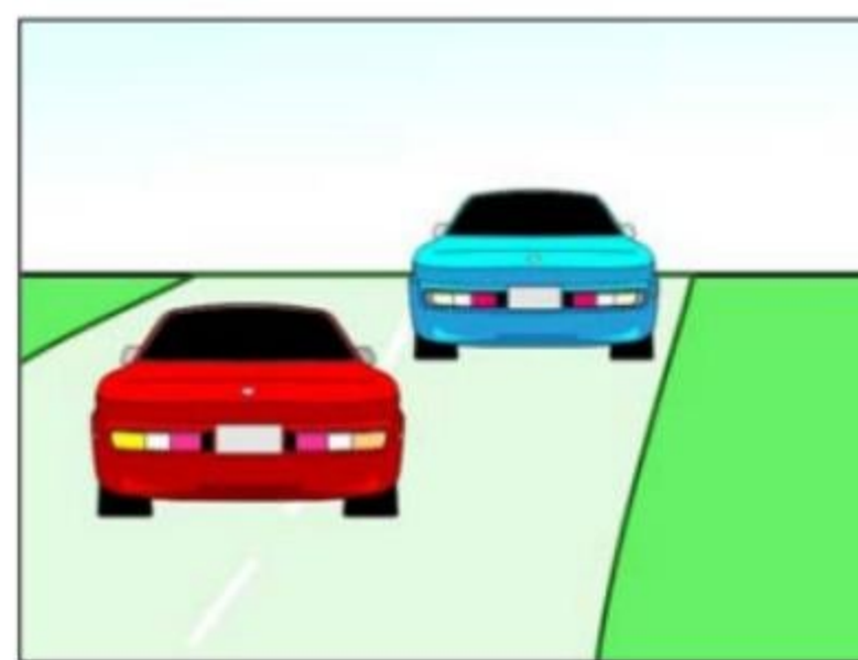
Мал. 75. Обгін автомобіля
