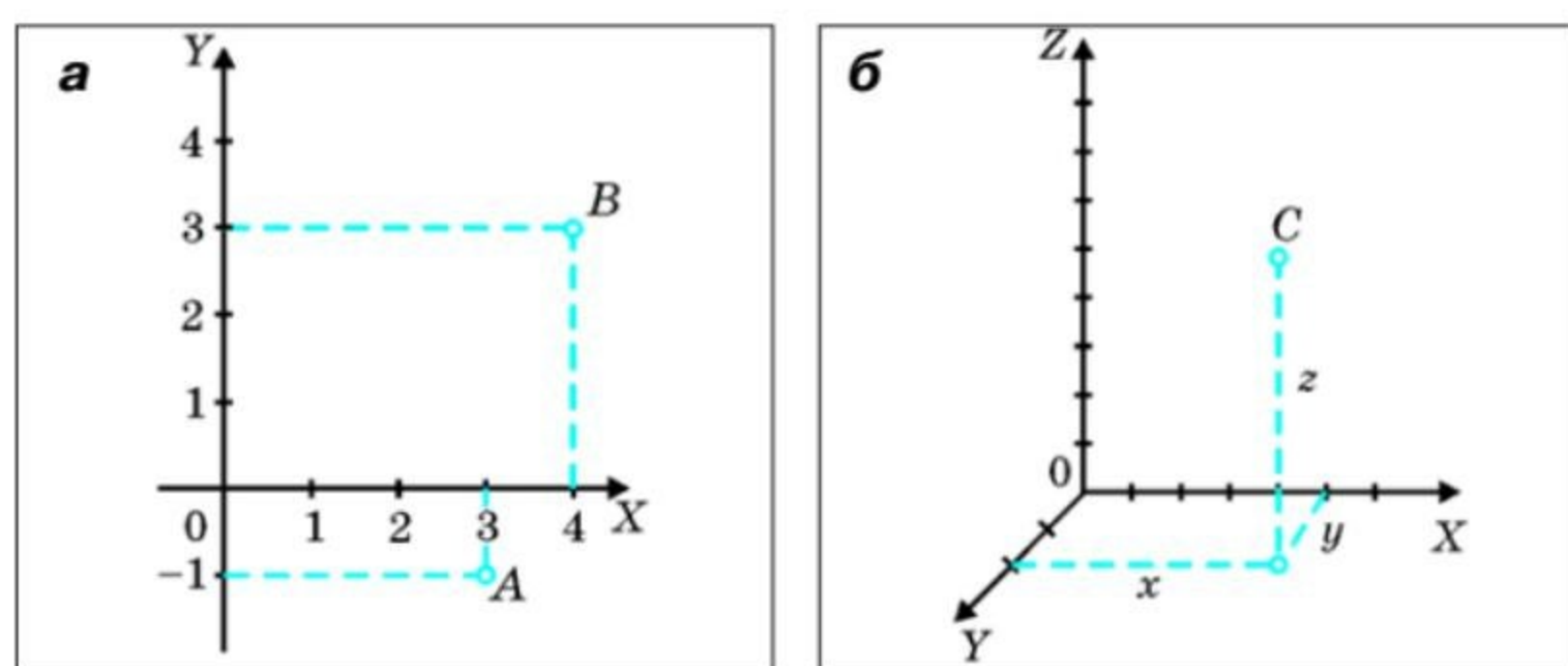
Мал. 29. Координати точки
