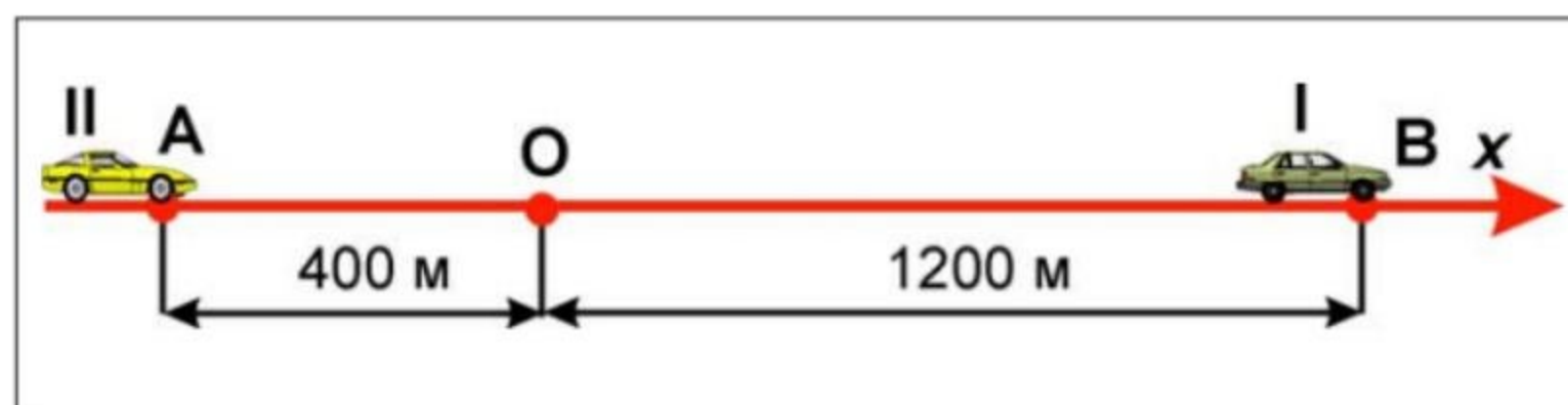
Мал. 28. До визначення положення тіла
