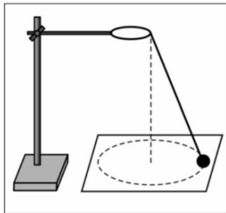
Мал. 45. При обертанні кульки тінь її коливається
