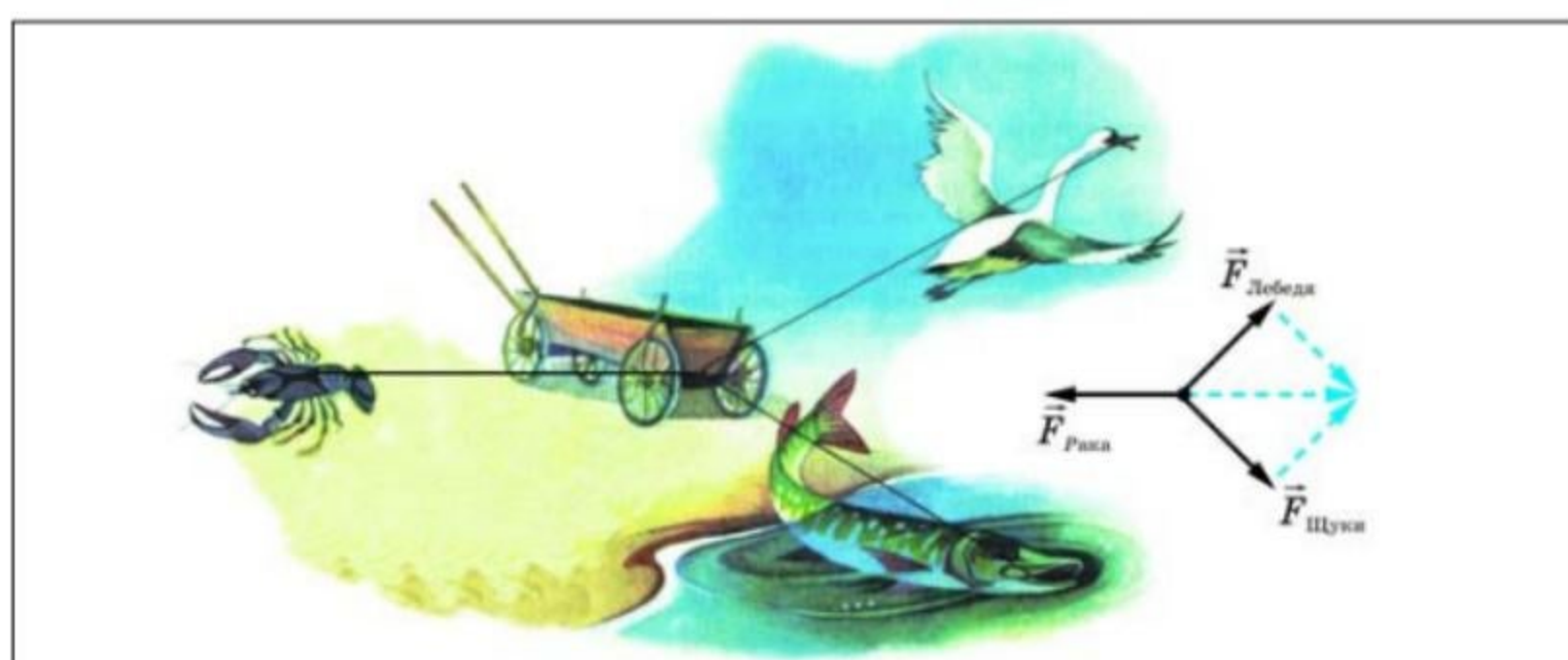
Мал. 83. Чому віз і «нині там»?
