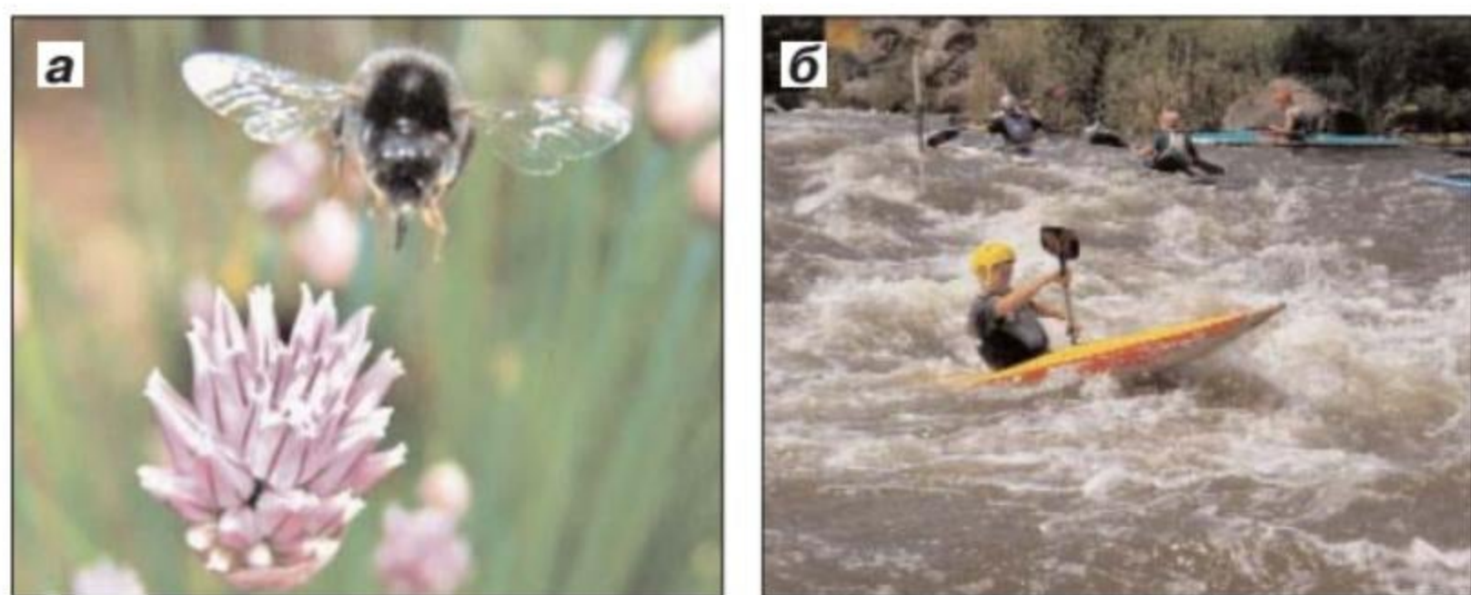
Мал. 24. Механічний рух
