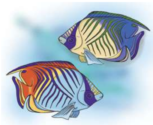
Хроматичні
