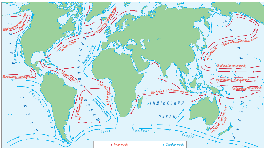
Мал. 1. Система кругообігів поверхневих течій Світового океану.
