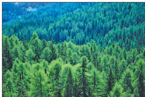
Мал. 3. Тайговий ліс на Алясці (США).
