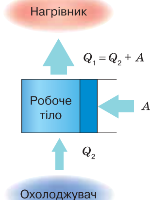
Мал. 71. Принцип дії холодильної машини
