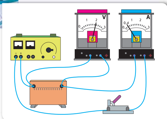
Мал. 153. Дослід зі встановлення залежності між силою струму й напругою: а — схема дослід; б — графічне представлення результатів дослід
