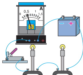
Мал. 160. Вимірювання сили струму в електричному колі з послідовним з'єднанням електроламп: а — між вимикачем і джерелом струму; б — між електролампами; в — між джерелом й електролампами
