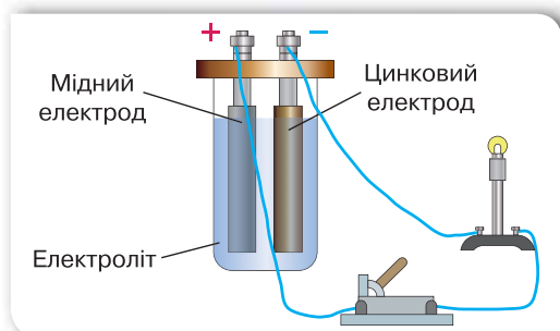
Мал. 126. Гальванічні елементи: а — принцип дії; б — різні види гальванічних елементів
