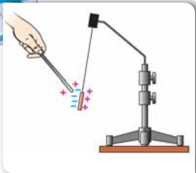
Мал. 107. Електризація через вплив
