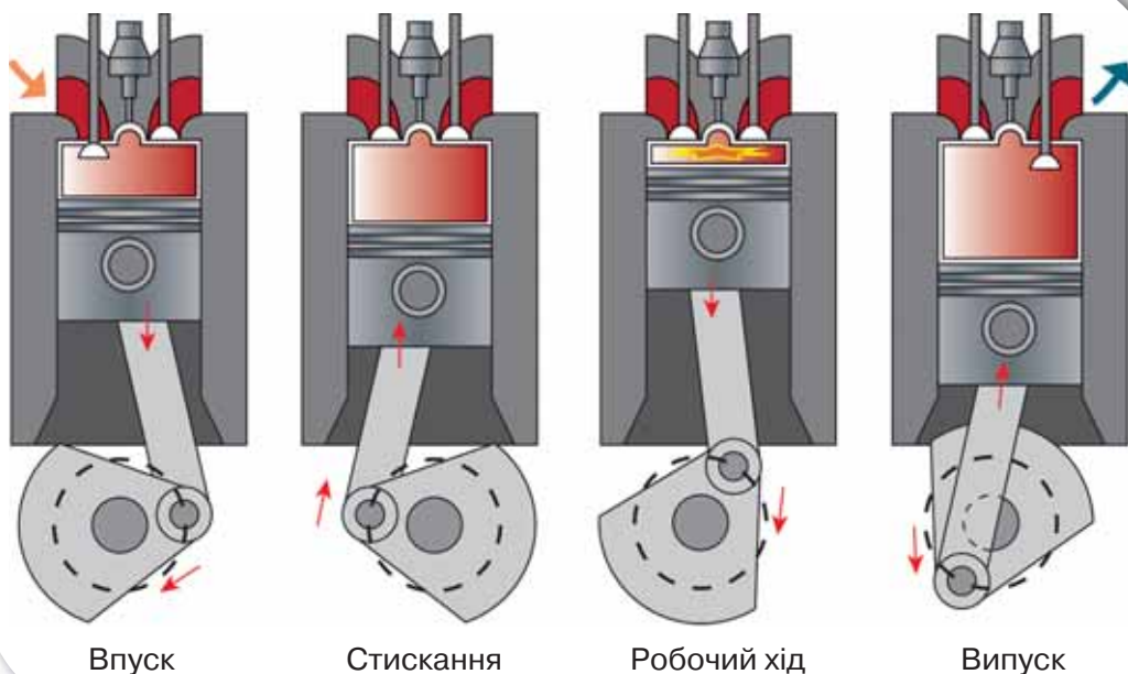
Мал. 66. Схема роботи чотиритактного ДВЗ
