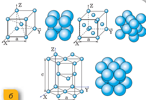
Мал. 17. Кристалічні тіла:
