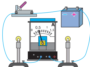
Мал. 160. Вимірювання сили струму в електричному колі з послідовним з'єднанням електроламп: а — між вимикачем і джерелом струму; б — між електролампами; в — між джерелом й електролампами
