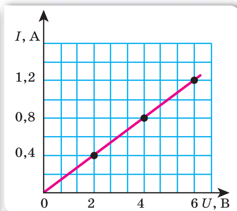
Мал. 153. Дослід зі встановлення залежності між силою струму й напругою: а — схема дослід; б — графічне представлення результатів дослід
