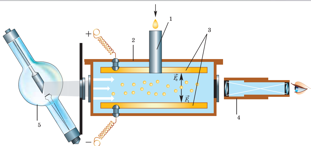
Мал. 116. Схема експериментальної установки дослідження Міллікена:
