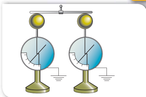
Мал. 115. Досліди з подільності електричного заряду: а — передача заряду одному з електрометрів; б — поділ електричного заряду
