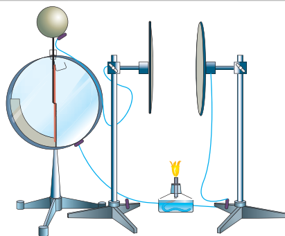
Мал. 203. Дослід з електропровідності повітря: а — за нормальних умов повітря не проводить електричний струм; б — нагріте повітря проводить електричний струм
