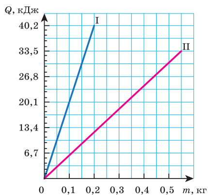
Мал. 48. Графіки залежності кількості теплоти від маси
