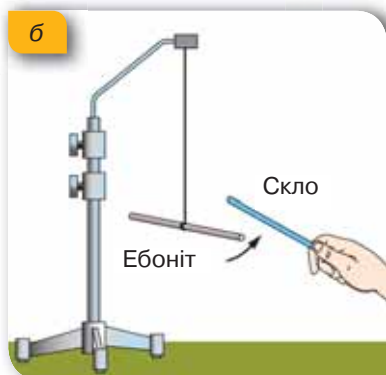
Мал. 88. Електромагнітна взаємодія: а — відштовхування; б — притягання
