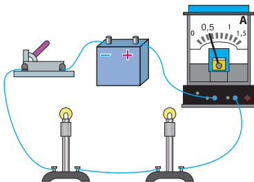
Мал. 160. Вимірювання сили струму в електричному колі з послідовним з'єднанням електроламп: а — між вимикачем і джерелом струму; б — між електролампами; в — між джерелом й електролампами
