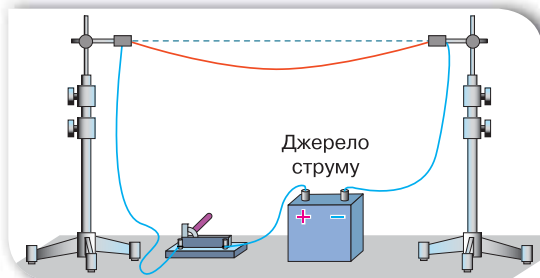
Мал. 131. Теплова дія струму
