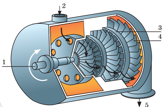
Мал. 68. Схема дії парової турбіни
