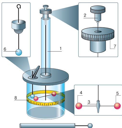
Мал. 118. Крутильні терези
