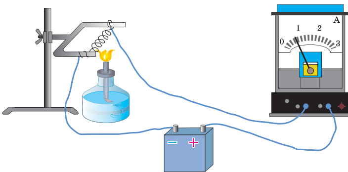
Мал. 196. Дослід, що демонструє залежність опору провідника від температури
