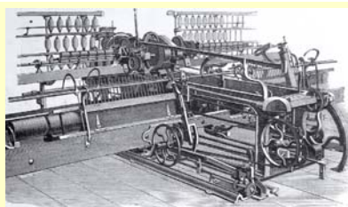
Механічний ткацький верстат, малюнок, 1775–1779 рр.
