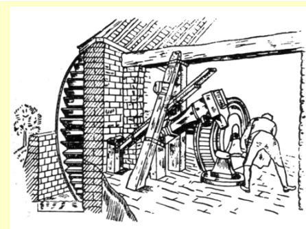
Ковальський молот із водяним приводом, XVIII ст.
