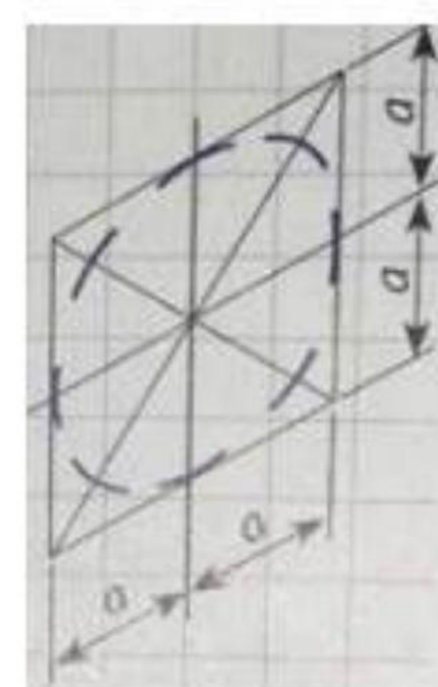
Побудова кола в ізометричній проєкції
