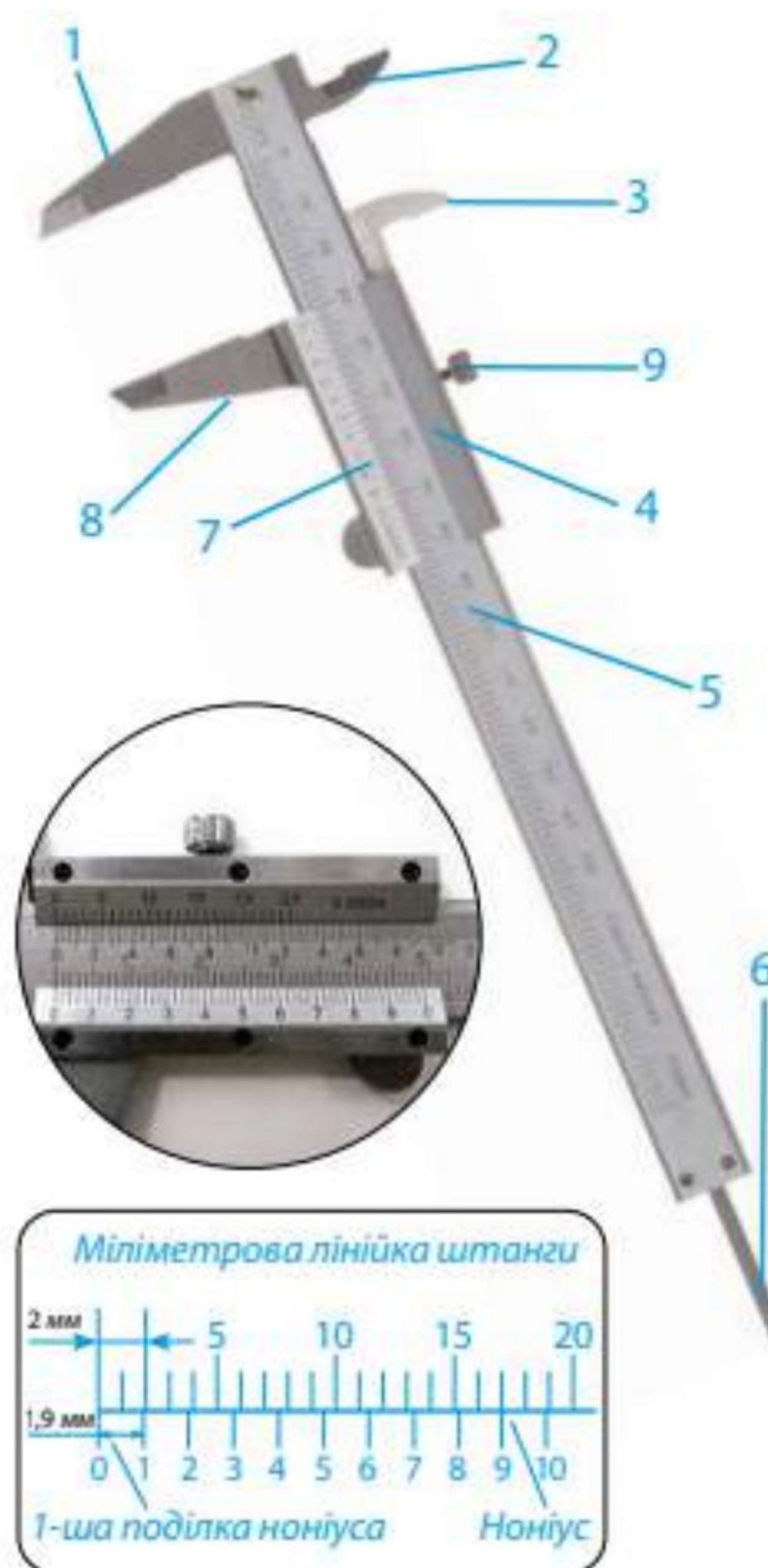
Мал. 132. Будова штангенциркуля і ноніус
