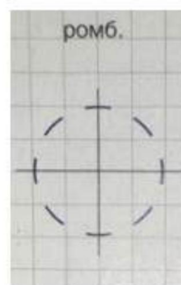
Побудова кола у фронтальній диметричній проєкції
