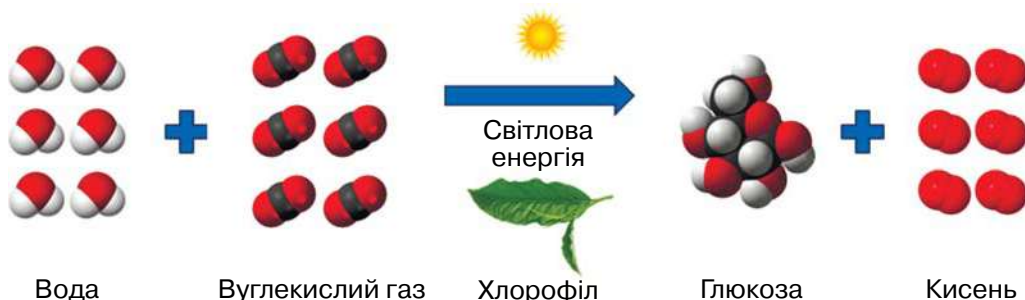
Мал. 11.7. Фотосинтез:
